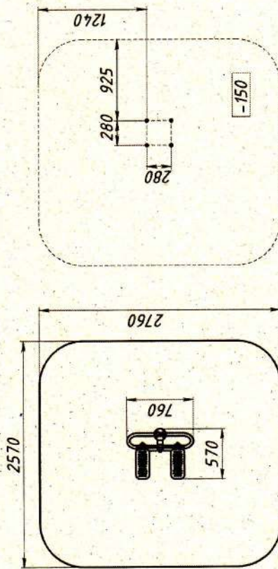
The equipment mounting plan (Схема монтажа оборудования)
